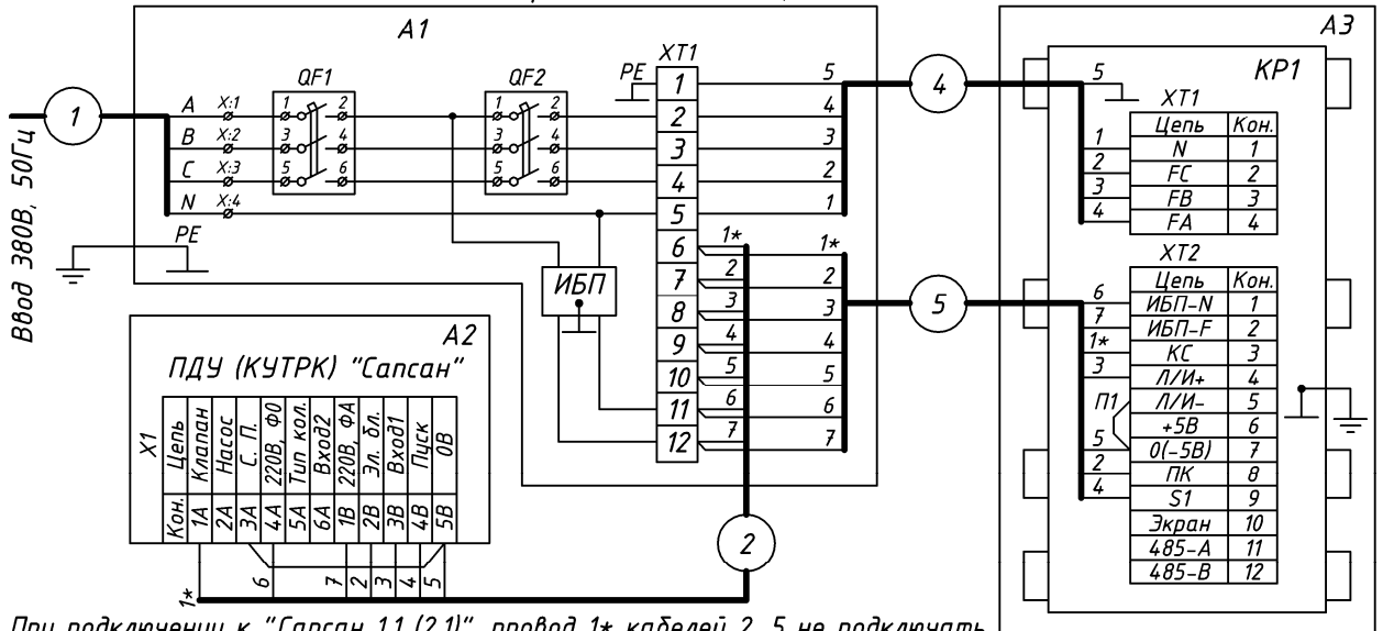
Рис. 2.2 Схема электрическая подключения ТРК "Квант-111" к ПДУ, КУТРК "Сапсан 2.1" (дискретность 0,01 л/имп)
