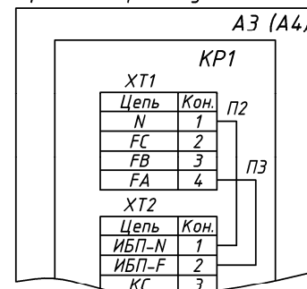
Рис. 1.2 Схема установки перемычек при отсутствии ИБП.
